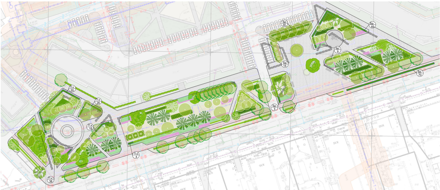
ПЛАН ПЕРЕСАДКИ М 1:500
